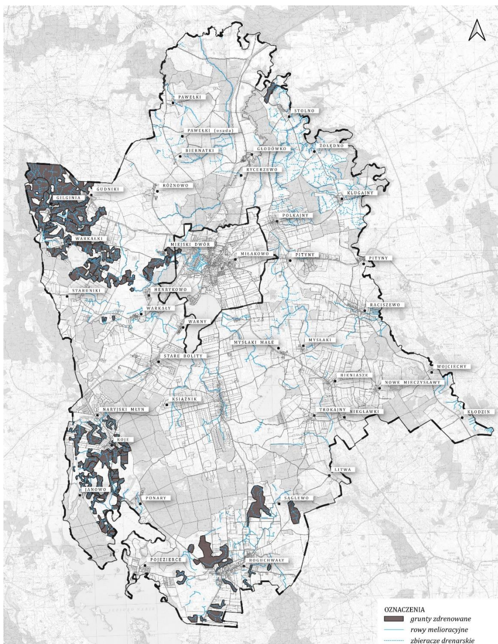
Rys.20. Grunty zdrenowane
